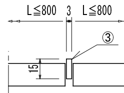
羽根分割要領 有効寸法ω
