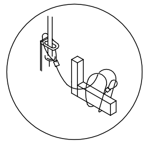
落下防止取付要領図
