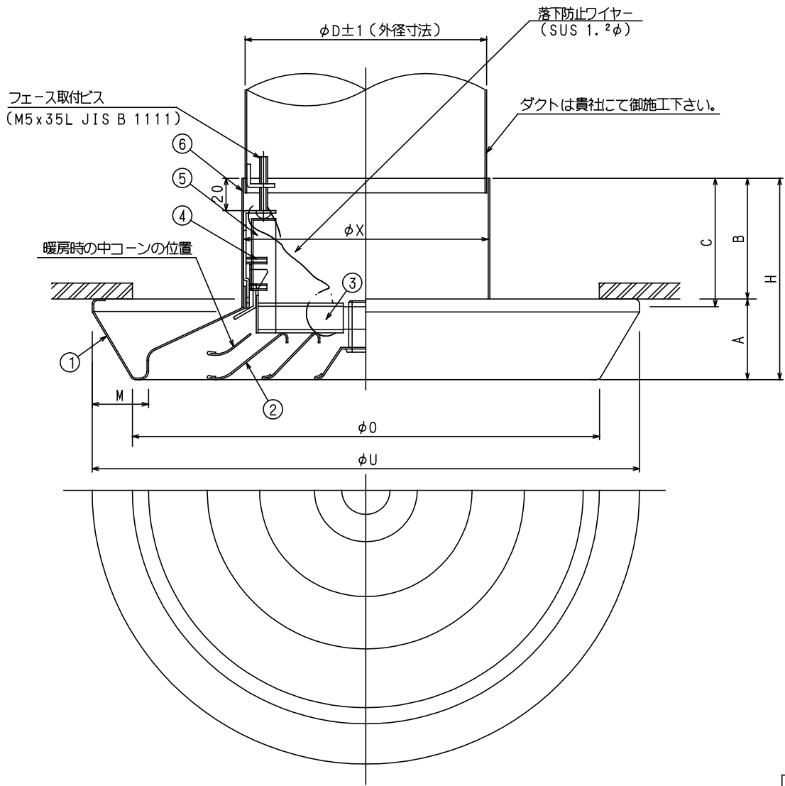
落下防止取付要領図
