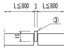
羽根分割要領 有効寸法 w \cdot h
