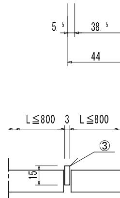
羽根分割要領 有効寸法 h
